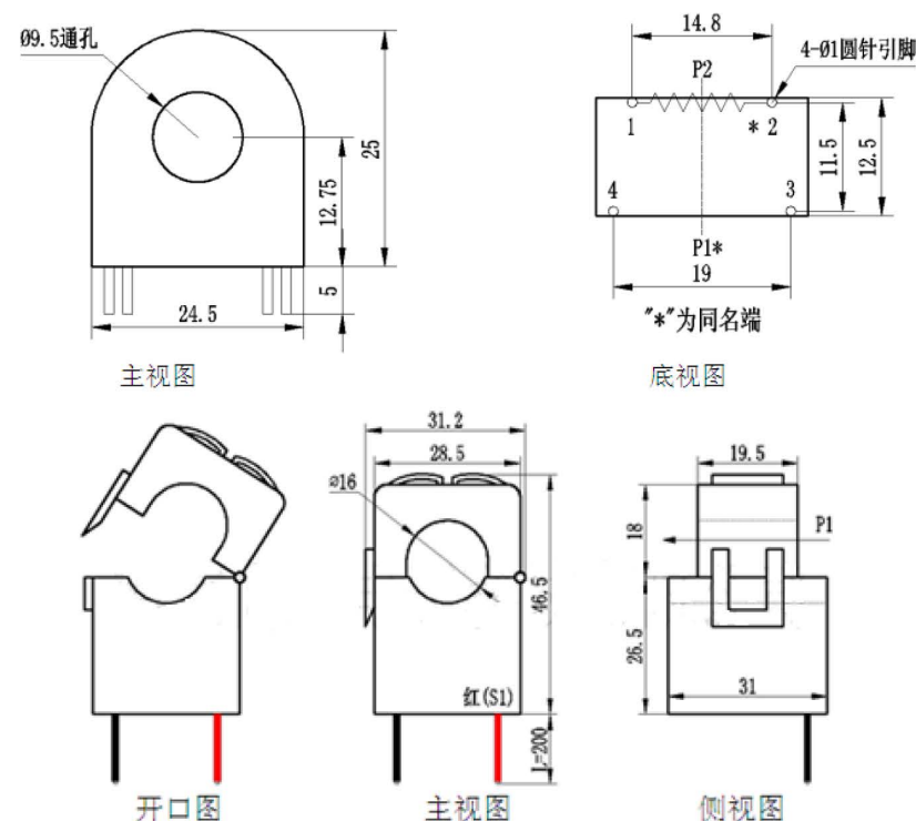
100A 开口式电流互感器外形尺寸图
