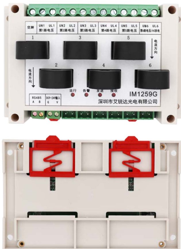
图 2.1 外形尺寸图（长 145x 宽 91x 高 58 单位：mm）
