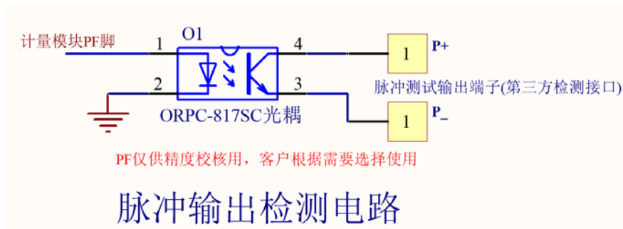
IM1281C 脉冲检测接口接线示意图
