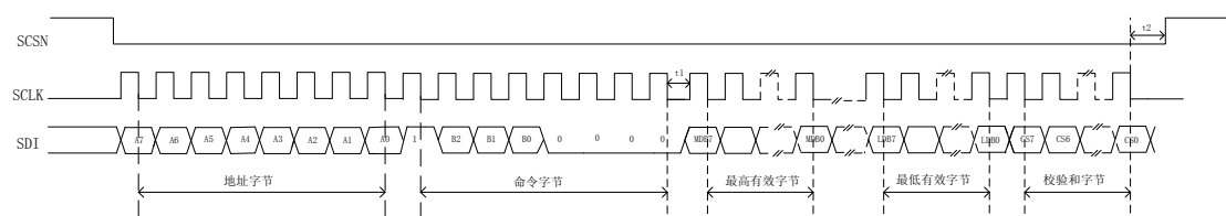
图 5-1 SPI 写时序
