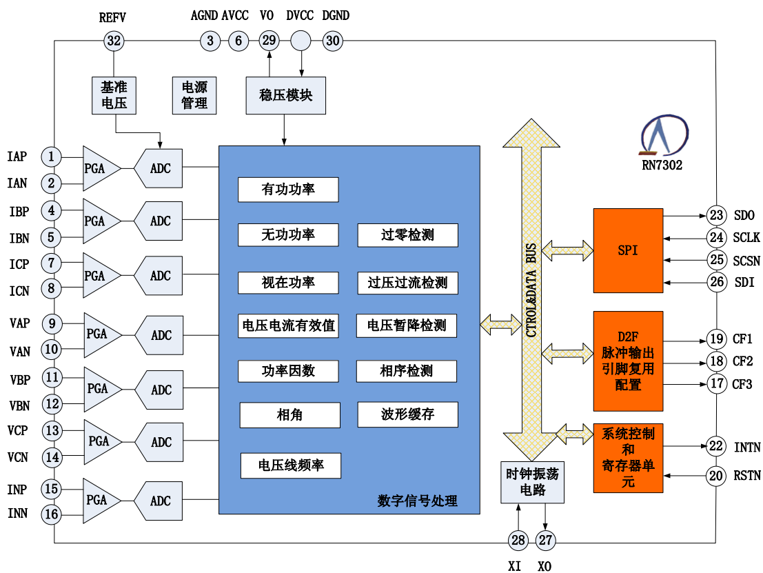
图 1-1 系统框图
