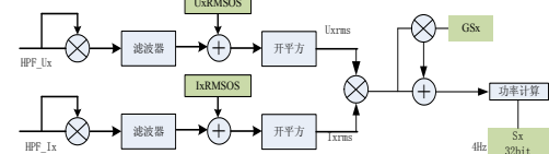
图2-3 分相视在功率
