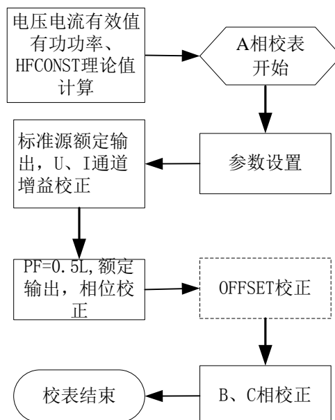
图4-1 校表流程
