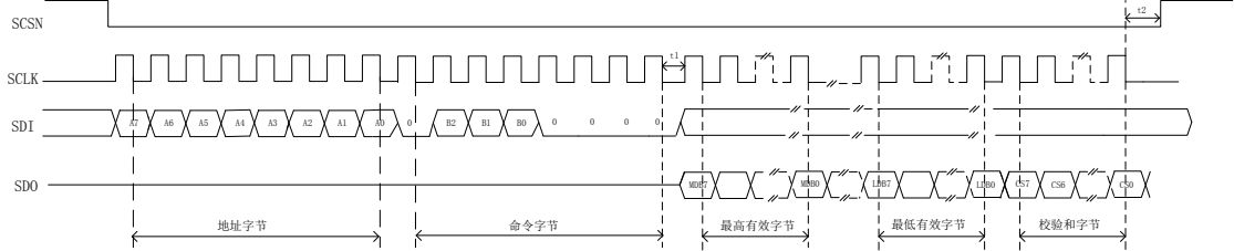
图 5-2 SPI 读时序
