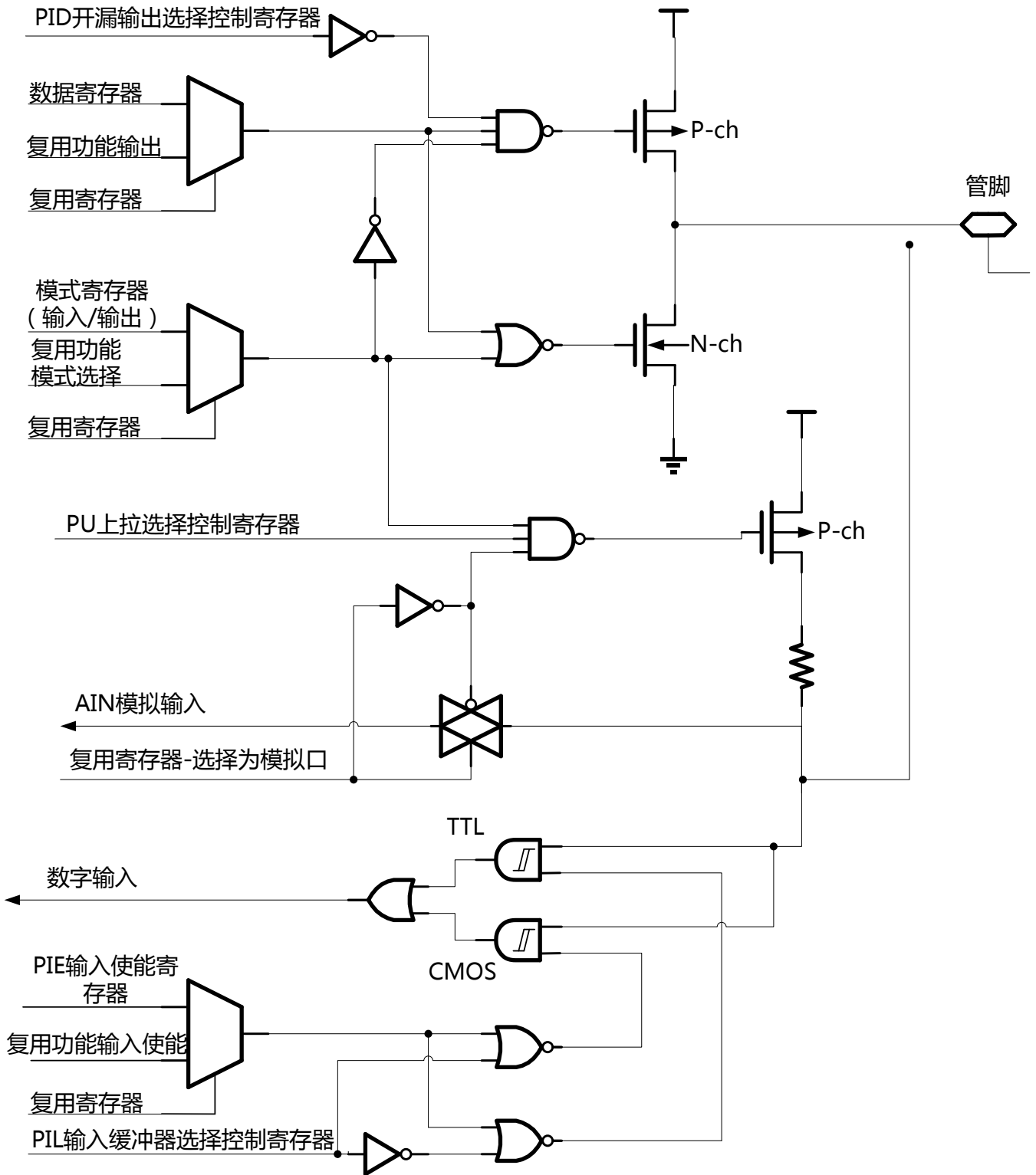
IO类型-PABULD3
