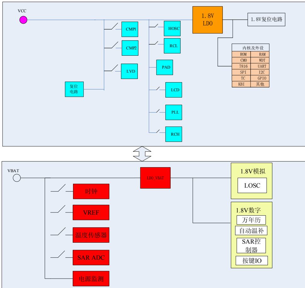
图 3.1 内部电源管理
