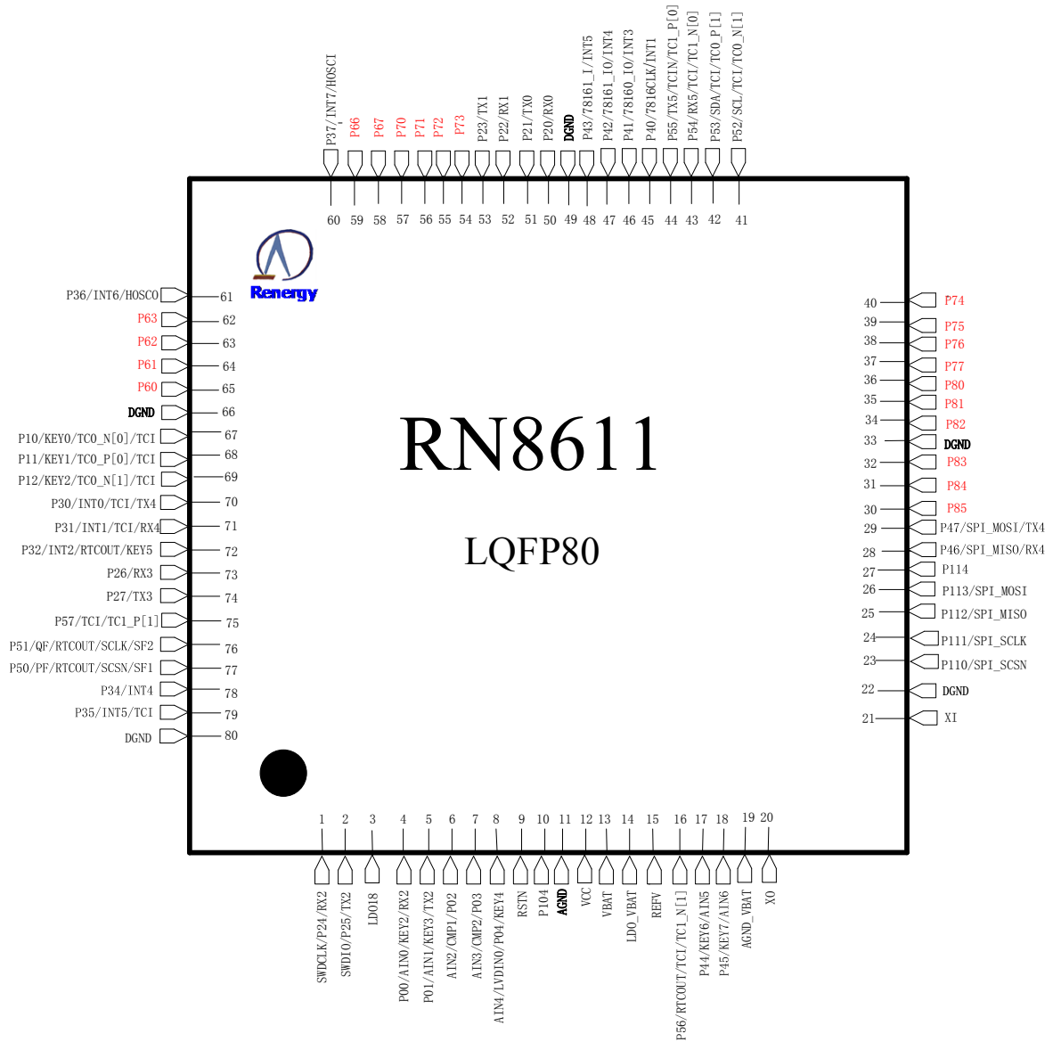
图 1.4RN8611 管脚排列图
