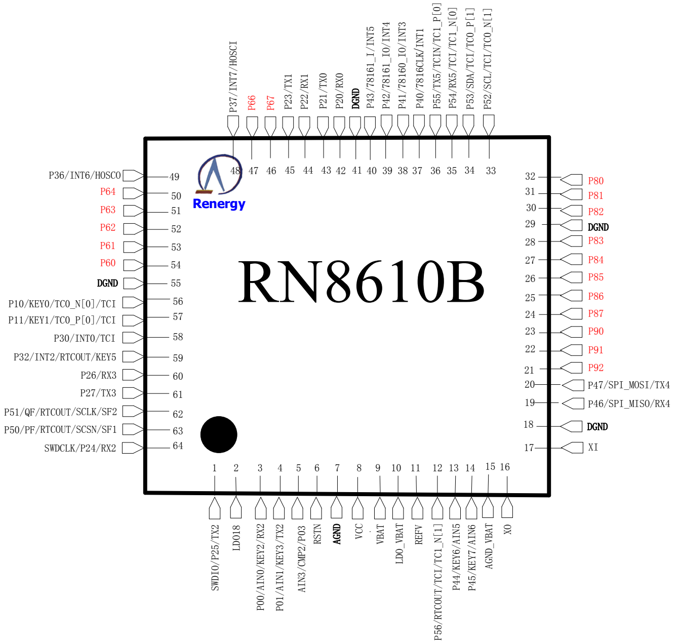
图 1.5 RN8610B 管脚排列图
